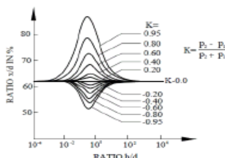
شکل پ - ت ۳- موقعیت مورد نیاز الکترودهای ولتاژ در یک زمین دو لایه
