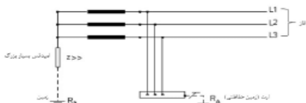
شکل پ - الف - ۵: سامانه اتصال زمین IT
