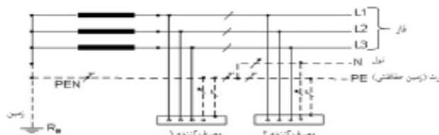
شکل پ - الف - ۳: سامانه اتصال زمین TN-C-S
