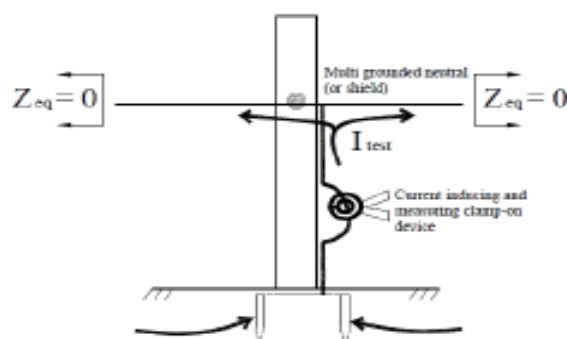
شکل پ - ت ۴- اندازه‌گیری مقاومت به روش کلمپی
