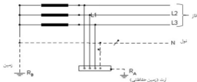
شکل پ - الف - ۴: سامانه اتصال زمین TT
