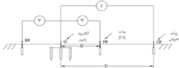
شکل پ-ت ۱- روش افت پتانسیل
