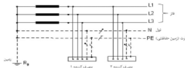
شکل پ - الف - ۲: سامانه اتصال زمین TN-S
