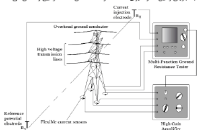
شکل پ-ت-۵- سامانه اندازه‌گیری مقاومت زمین دکل با استفاده از روش افت پتانسیل و اندازه‌گیری‌های جریان ناشی
