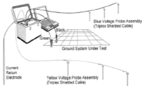
شکل پ-ت ۶- اندازه‌گیری امپدانس زمین با استفاده از مالتی-متر زمین کامپیوتری
