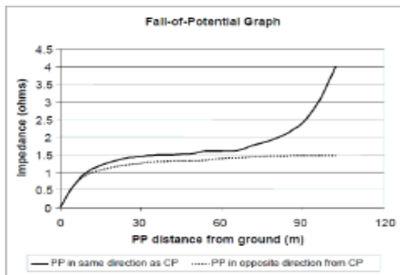
شکل پ-ت ۲- امیدانی به نسبت فاصله پراب ولتاژ برای روش افت پتانسیل
